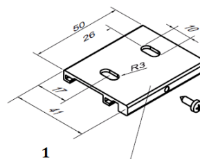
1. Klip montażowy
